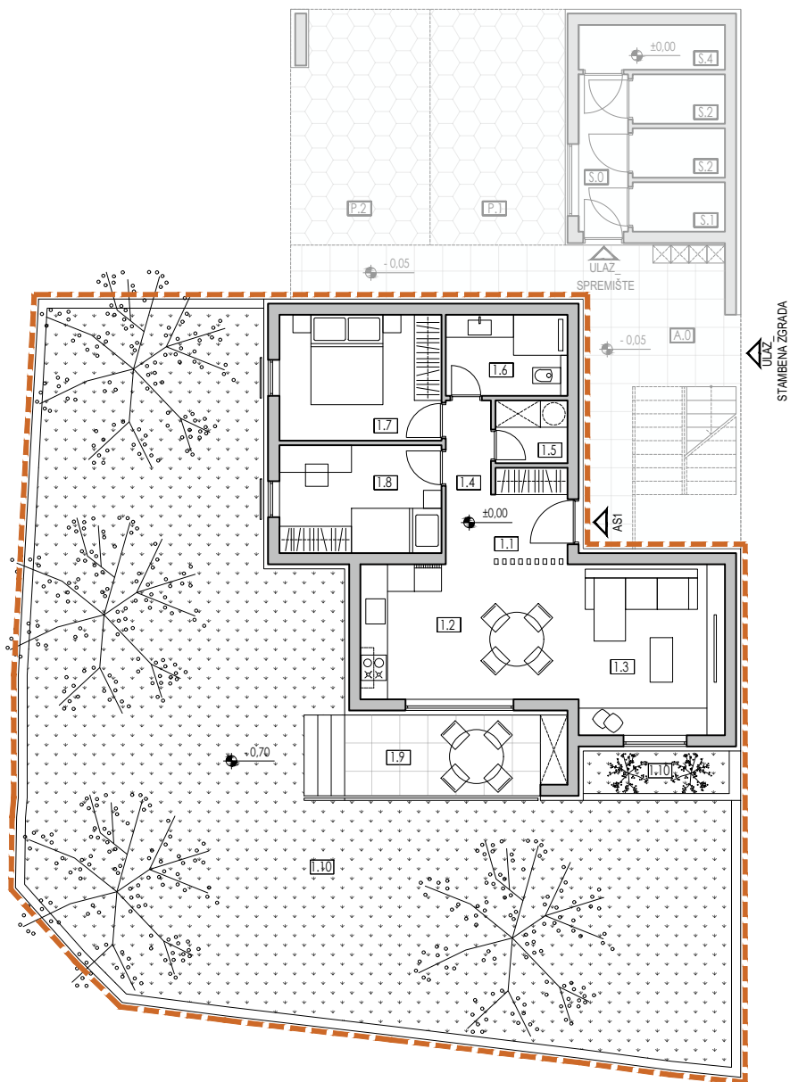
_tlocrt prizemlja _m1:150
