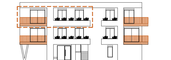
_južno pročelje
