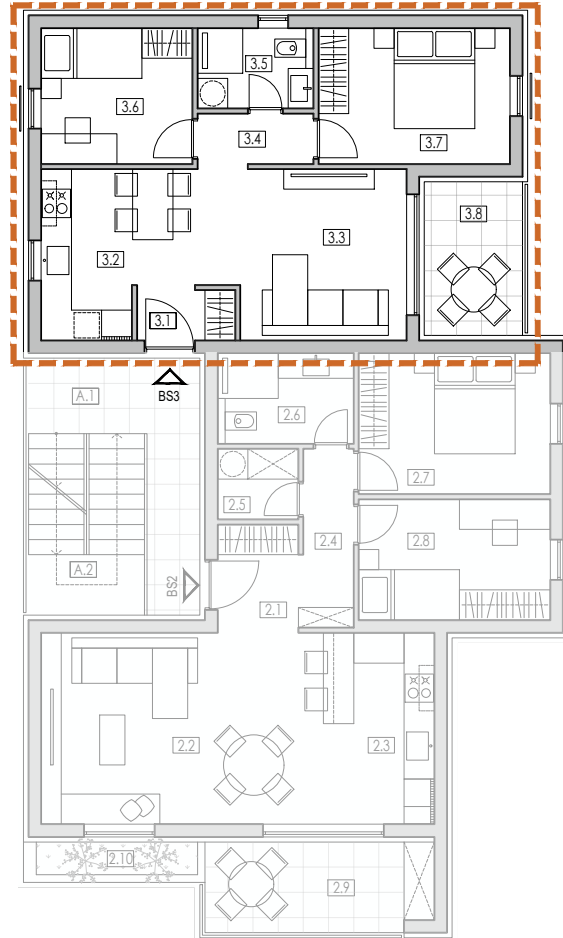
_tlocrt 1.kata_m1:150
